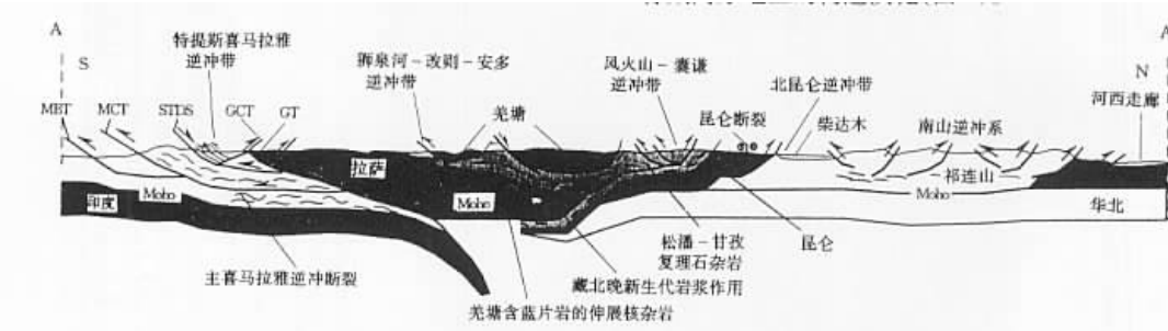
图 3 横跨喜马拉雅-青藏高原造山带的地质剖面示意图
