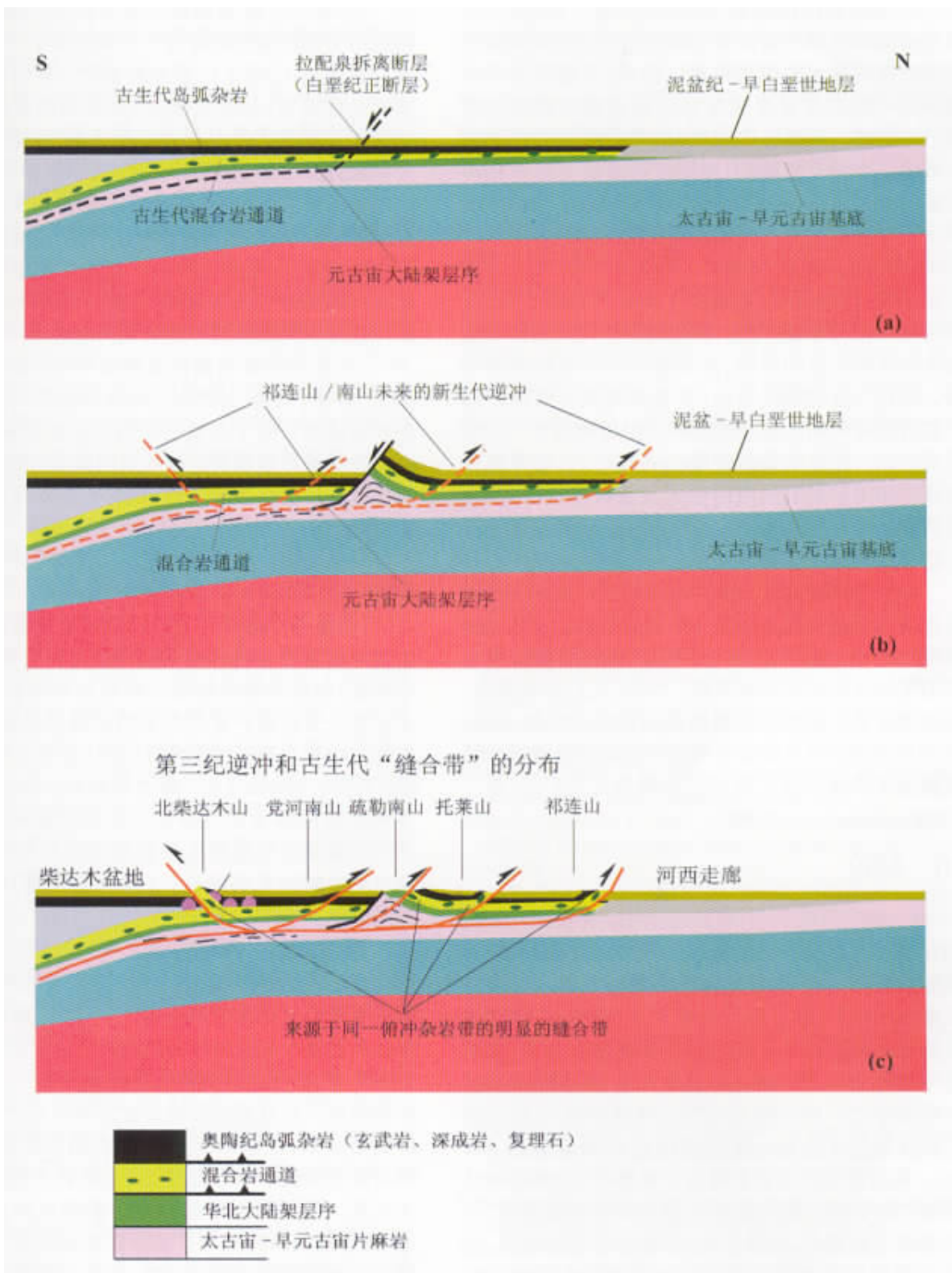
图 8 拉配泉和祁连山地体新生代变形前的构造地层断面
