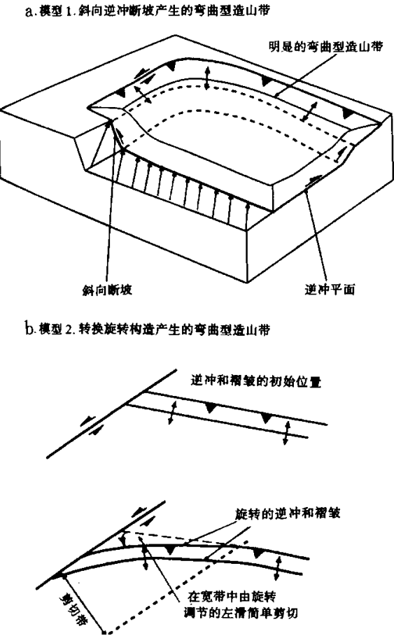
图 6 沿阿尔金断裂系构造弯曲线状带的对比模型
