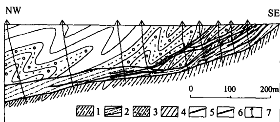
图4 210 金矿床 0 线地质剖面图
