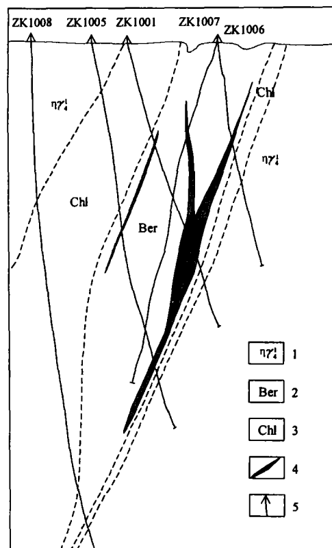
图5 金窝子金矿床10线地质剖面(据有色704队资料)
