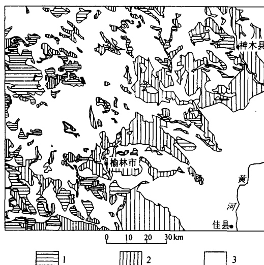
图3 沙漠化土地发展趋势图
