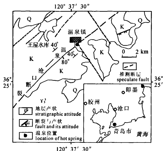
图1 青岛即墨温泉位置及地质略图
