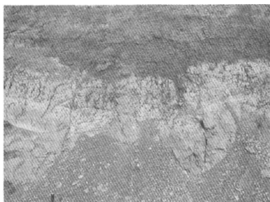
图4 温泉盆地对冲式第四纪以来活断层
