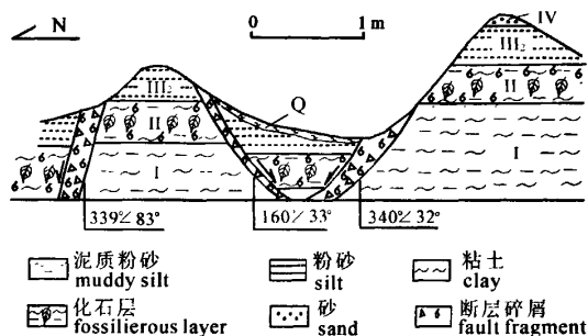
图2 温泉盆地堑—垒型第四纪以来活断层剖面图
