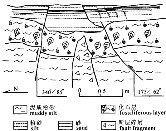
图3 温泉盆地对冲式第四纪以来活断层剖面图
