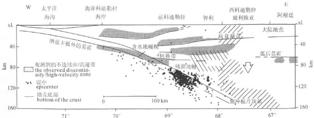
图 12 横过科迪勒拉山地球物理剖面解释
