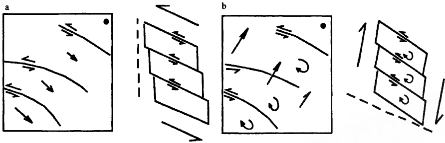
图 8 单剪切-旋转模式示意图
