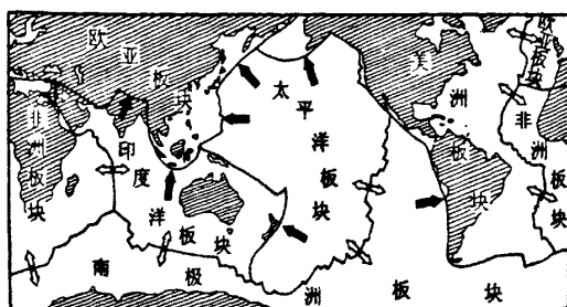
图 6 全球六大岩石圈板块划分图(据勒皮雄, 1968)
