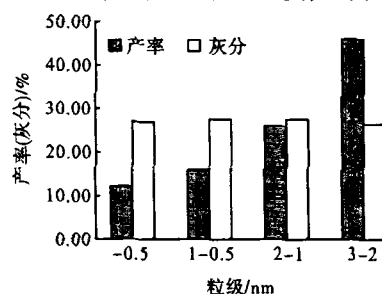
图1 煤样筛分试验结果
