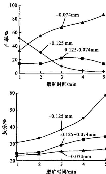
图2 不同磨矿时间下各粒级产率和灰分的变化曲线
