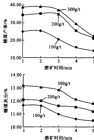
图4 “一粗一精”浮选试验结果
