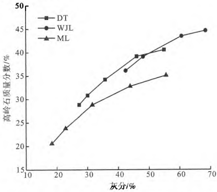
图 6 尾煤累计灰分—高岭石累计含量关系曲线
