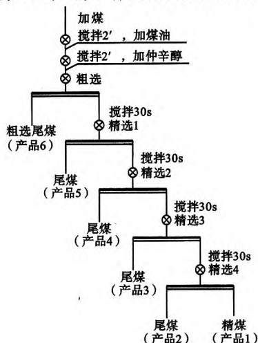
图2 浮选试验流程
