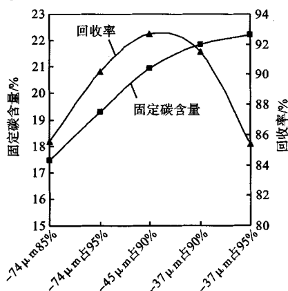
图1 磨矿细度对粗精矿指标的影响
