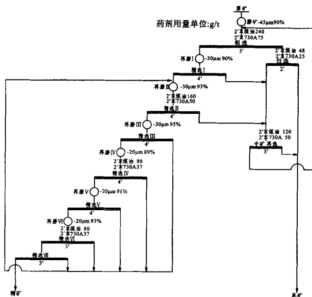
图 6 闭路试验流程
