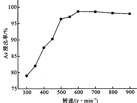
图4 搅拌速度对白烟尘浸出的影响
