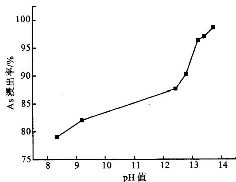
图1 pH 值对白烟尘浸出的影响
