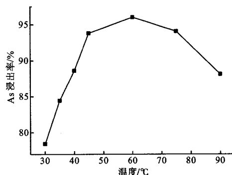
图3 浸出温度对白烟尘浸出的影响
