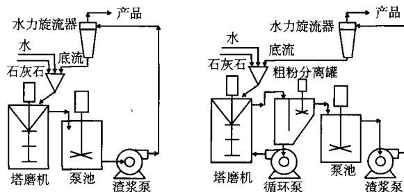
左 - 不含粗粉分离罐的单闭路
