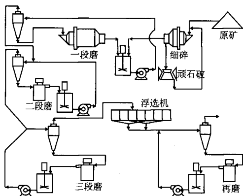
图1 选矿厂常见碎磨工艺流程
