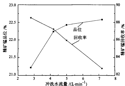
图5 强磁选机冲洗水流量实验结果
