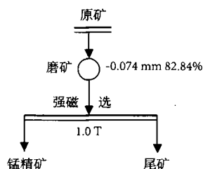
图2 磁选实验流程
