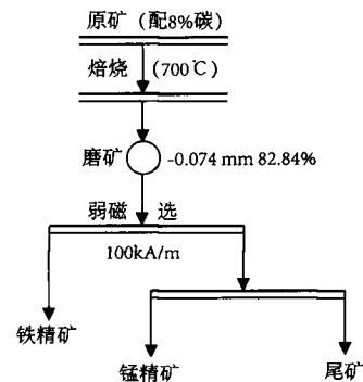
图 1 磁化焙烧锰铁分离实验流程
