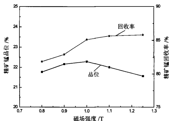
图4 磁选强度条件试验结果
