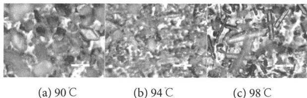
图 3 不同反应温度下的晶体形貌
