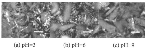
图 5 不同 pH 值时的晶体形貌
