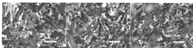
图 4 不同固液比下的晶体形貌
