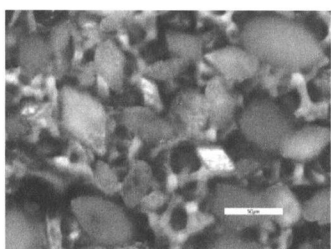
图 1 脱硫石膏晶貌
