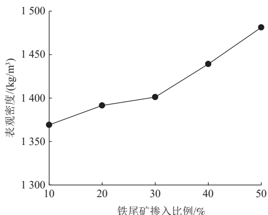
图3 表观密度和铁尾矿占比的关系
