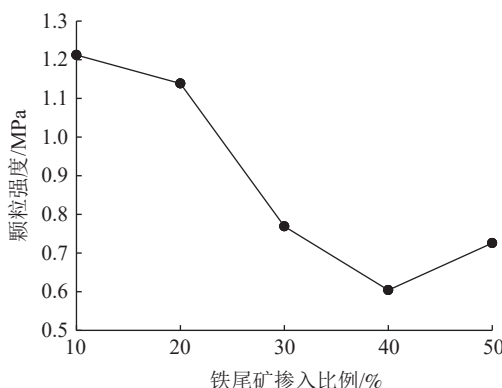
图5 颗粒强度和铁尾矿占比的关系
