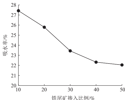
图4 吸水率和铁尾矿占比的关系
