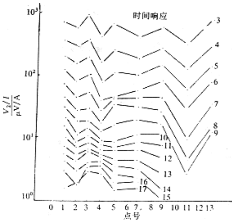
图3 150线TEM剖面(据蒋慎君资料)
