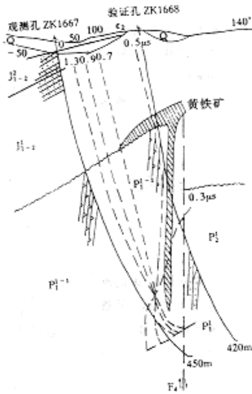
图3 150线TEM剖面(据蒋慎君资料)
