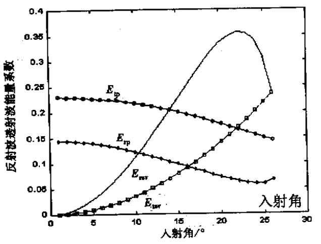
图 3 不同入射角反射波透射波能量系数
