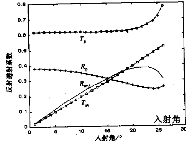
图 2 不同入射角位移反射透射系数
