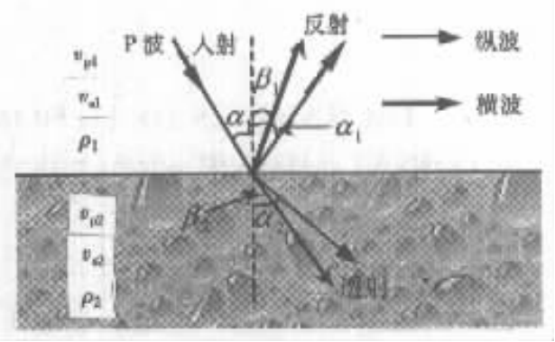
图 1 弹性波在两层结构分界面反射折射示意 \rho_2 表示。假定两个半空间在界面处紧密接触 ,
