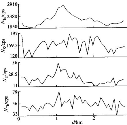
图 2 新疆某地航空放射性测量异常剖面
