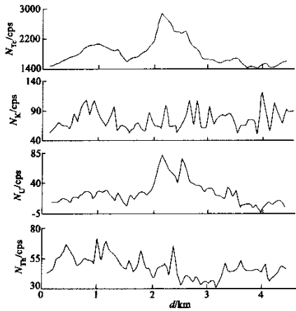
图 1 云南某地航空放射性测量异常剖面 步浓缩,炉渣中放射性强度较高,炉渣大量堆积,并用来制成砖坯构筑围墙及房屋,造成了大片的放射性污染区域。现场利用 GR-410 多道伽马能谱仪(碘化钠晶体,体积 347 cm 3 )在较平坦的堆场进行测量(表 1)。测得铁矿石钾、铀、钍含量分别为 0.34%、 12.2 \times 10^{-6} 、 4.7 \times 10^{-6} ,空气吸收剂量率(D)为 85.7 nGy/h 测得废渣中钾、铀、钍含量分别为 0.39%、 33.8 \times 10^{-6} 、 15.8 \times 10^{-6} ,空气吸收剂量率 236.3 nGy/h。废渣制砖构成的墙体钾含量最高达 0.55%,
