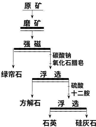
图 1 硅灰石矿除杂原则流程
