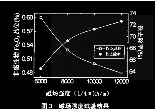
图 3 磁场强度试验结果
