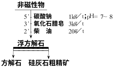
图 4 浮选分离方解石工艺条件
