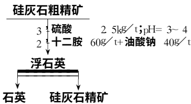
图 5 浮选分离石英试验工艺条件
