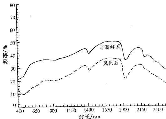
图4 花岗片麻岩反射光谱
