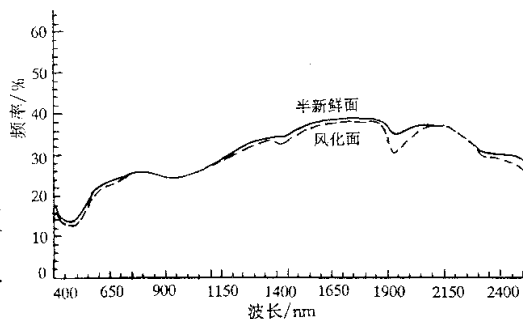
图3 红旗营子群黑云母斜长片麻岩反射光谱
