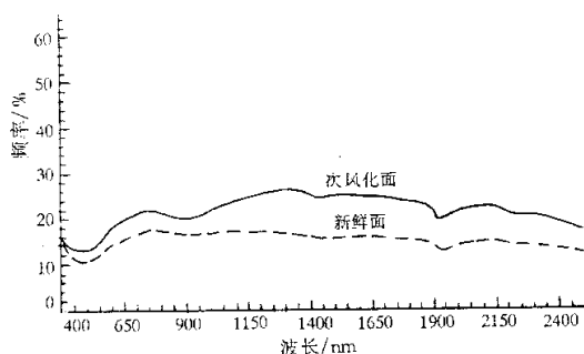
图2 侏罗系张家口群流纹岩反射光谱
