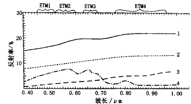
图 1 新疆焉耆—博斯腾湖一带几种土壤及湖水反射光谱曲线
