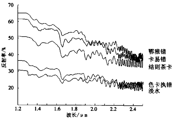
图1 湖泊波谱曲线图
