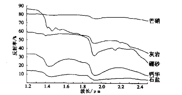
图 2 固体盐类波谱曲线图 波段均为一条直线,其中硼砂在可见光波段反射率高,在近红外波段反射率低;芒硝在可见光和近红外波段反射率相近,变化较小,而石盐介于二者之间。采用 TM2/TM7 比值图像区分 3 种矿物,取得了满意效果。具体方法是:将 TM2 和 TM7 波段数据
