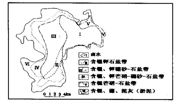
图 3 扎不耶茶卡南湖盐类沉积分带图 比,发现白色代表硼砂或以硼砂为主,红色代表石盐或以石盐为主,绿色代表芒硝或以芒硝为主。为了检验判断结果的正确性,本次选择工作程度低、找矿潜力大的已知盐湖鄂雅错、才玛尔错和未开展过工作的找矿靶区纳屋错、查哈那泊等 6 个盐湖进行了验证,部署了浅井工程并取样分析,结果和实际情况基本相符。其中预测的纳屋错芒硝找矿靶区经验证为一大型芒硝矿床。
