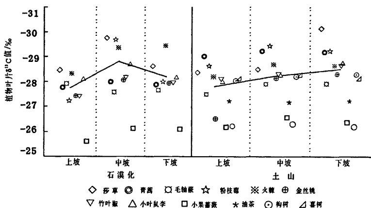
图3 不同坡位间植物叶片 \delta^{13}\text{C} 值
