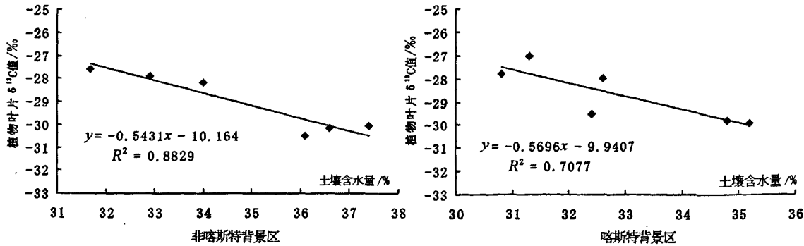
图5 不同背景区植物叶片 \delta^{13}\text{C} 值随土壤含水量的变化趋势
