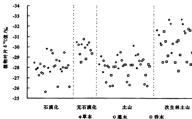
图2 不同样地植物叶片 \delta^{13}\text{C} 值散点图
