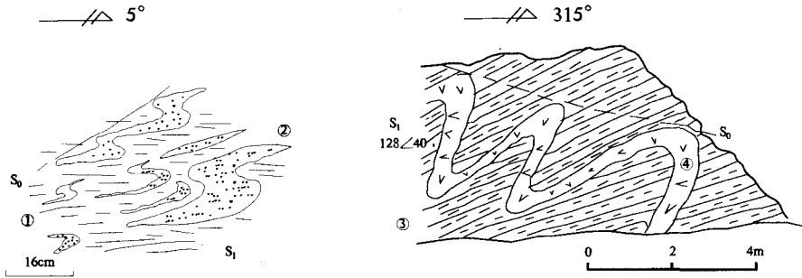
图2 石碌群中的顺层剪切面理
