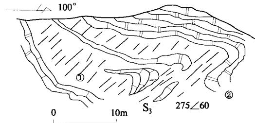
图4 石碌群北一铁矿中的 S_3 劈理
