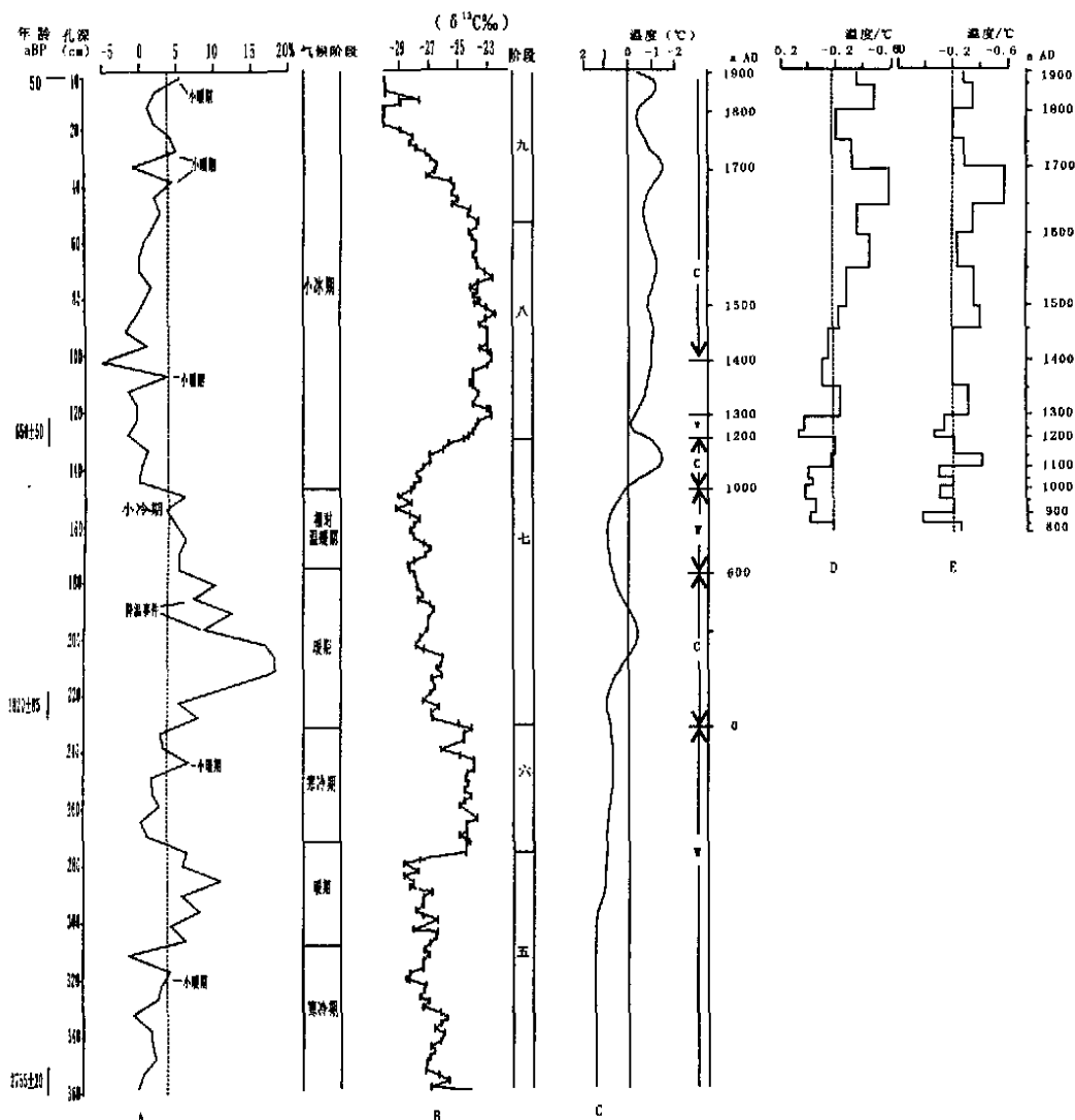
图2 ZK01 钻孔约 2760a BP 以来孢粉 I 值变化曲线对比图
