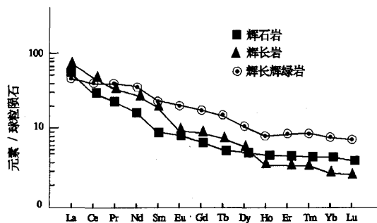
图 2 岩体稀土元素分配图
