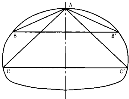
图 2 洞内测桩布置图
