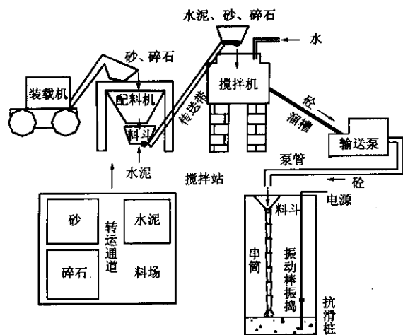
图1 泵送砼浇筑流程图
