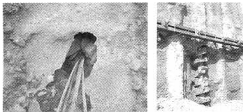
图1 完成的部分锚固孔
