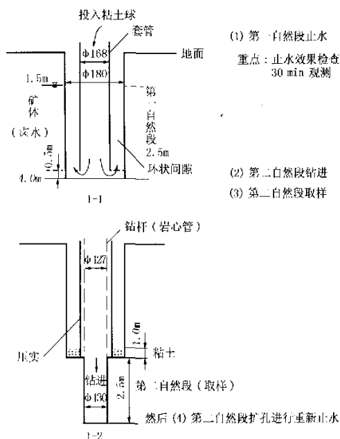
图 1 地质勘探孔分段止水示意图
