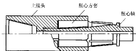
图1 倒扣接头结构示意图
