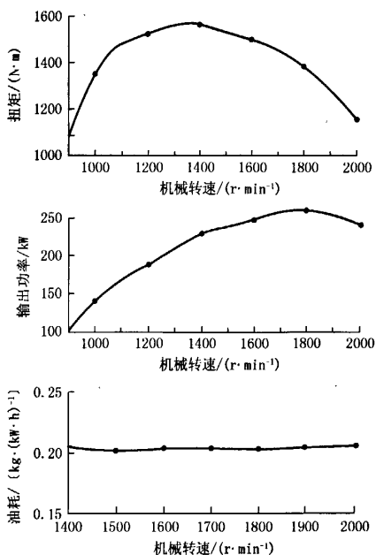
图 2 QSL9 柴油机外特性曲线
