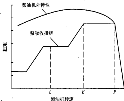
图3 发动机与液压泵功率匹配曲线
