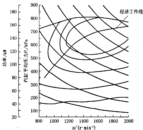
图 1 柴油机万有特性曲线
