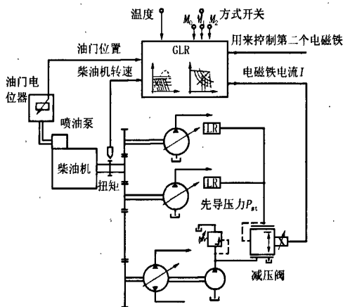
图4 GLR控制器的液压回路示意图
