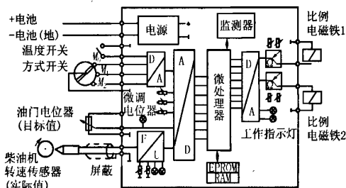
图5 GLR控制器的电路示意图
