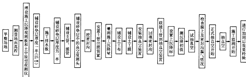
图1 施工工艺流程图
