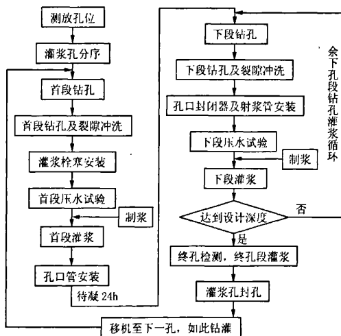
图1 帷幕灌浆施工工艺流程
