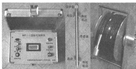
图 3 QXY-II 型钻孔倾斜仪
