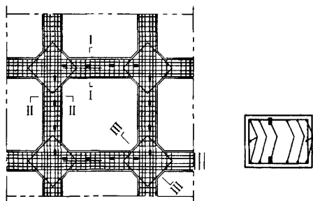
图 11 钢筋应力计埋设示意图
