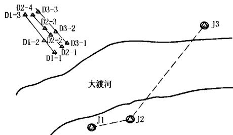
图9 地表大地变形监测布置图
