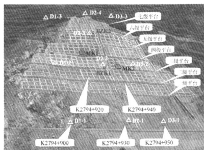
图8 监测设施布置图
