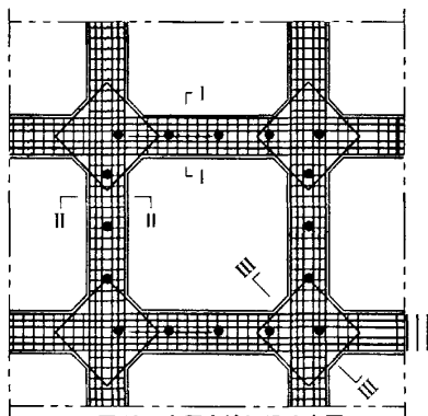
图 10 土压力计埋设示意图
