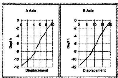
图 6 sjb2-2 号钻孔深部位移图
