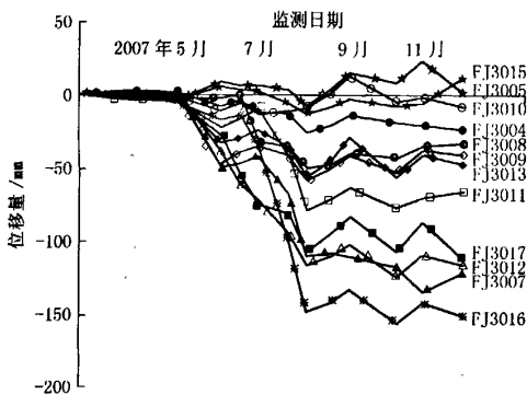
图 4 各测点垂直方向位移矢量曲线
