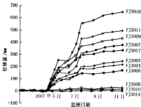
图 2 各测点正北方向位移矢量曲线
