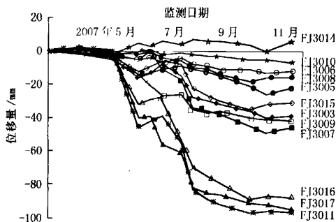
图 3 各测点正东方向位移矢量曲线
