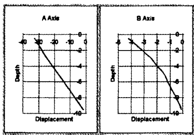
图 5 sjb2-1 号钻孔深部位移图
