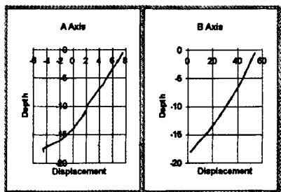
图 7 sjb2-3 号钻孔深部位移图
