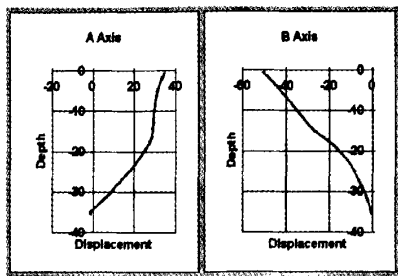
图 8 sjb2-4 号钻孔深部位移图
