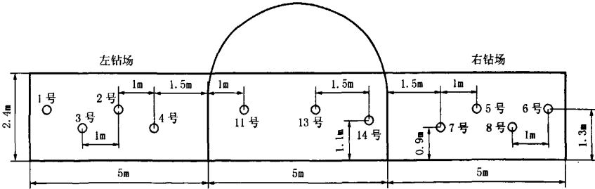
图 1 钻孔布置断面示意图
