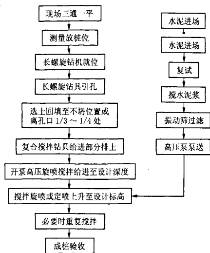
图1 旋喷搅拌水泥土桩止水帷幕施工工艺流程图
