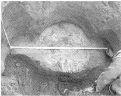
图4 成桩效果图
