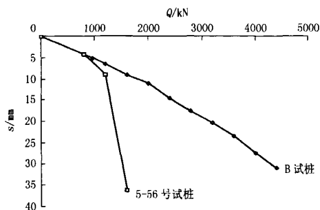
图5 虹桥路北陈家行、金牌大厦试桩 Q-s 曲线(二)
