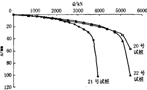
图 2 金山石化涤纶二厂试桩 Q-s 曲线
