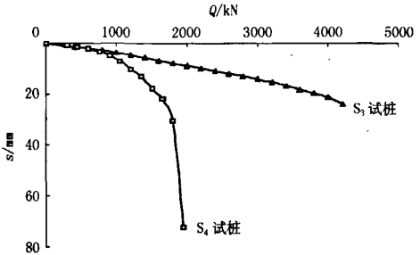
图 1 金山石化塑料厂试桩 Q-s 曲线
