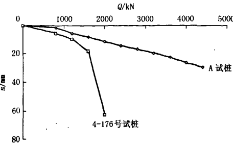
图 4 虹桥路北陈家行和金牌大厦试桩 Q-s 曲线(一)
