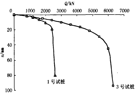
图 3 奉贤 728 工程试桩 Q-s 曲线
