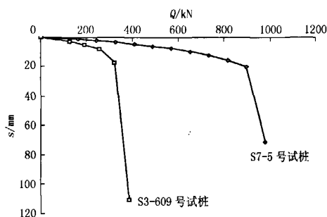
图6 青浦赵巷某工地试桩 Q-s 曲线
