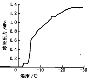
图 17 测温孔 2 与测压孔 3 温度 - 冻胀压力曲线
