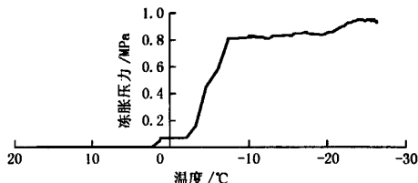
图 16 测温孔 3 与测压孔 1 温度 - 冻胀压力曲线
