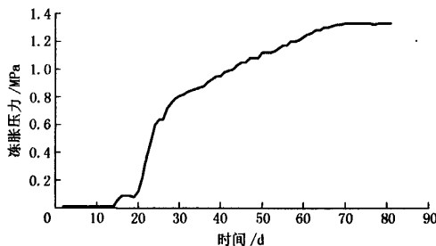
图 15 测压孔 3 测点 1 冻胀压力曲线
