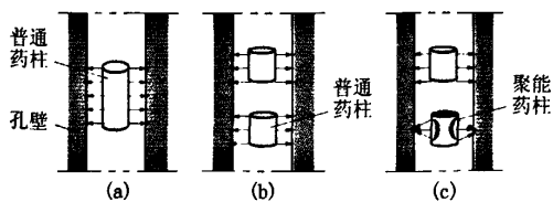
图 1 孔内局部岩石爆破破碎加载形式
