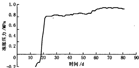
图 14 测压孔 1 测点 2 冻胀压力曲线
