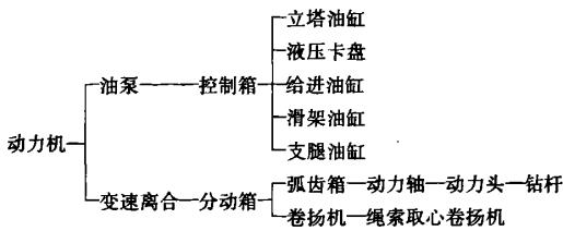
图1 XL-5型钻机传动路线图
