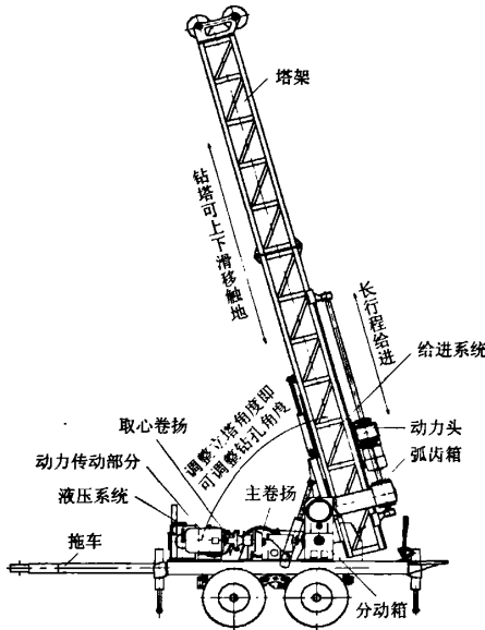
图2 XL-5型钻机结构示意图
