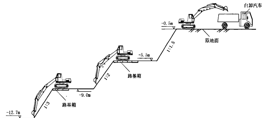
图 1 基坑开挖纵断面
