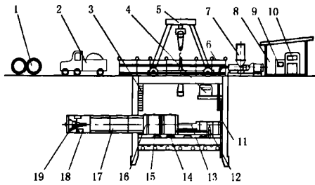
图1 顶管施工设备简图
