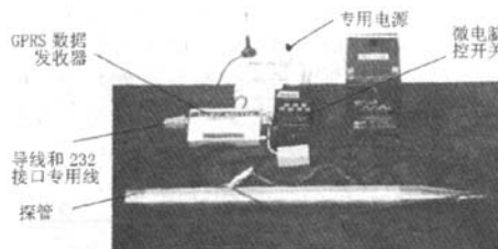
图7 CZ-2 型钻孔倾斜仪全套设备示意图
