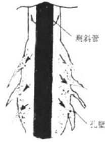
图 3 固结水泥流失测斜管松动示意图
