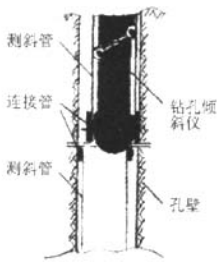
图 1 测斜管被剪断不能下测示意图
