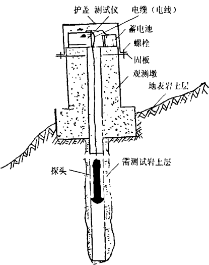
图 13 现场测试示意图
