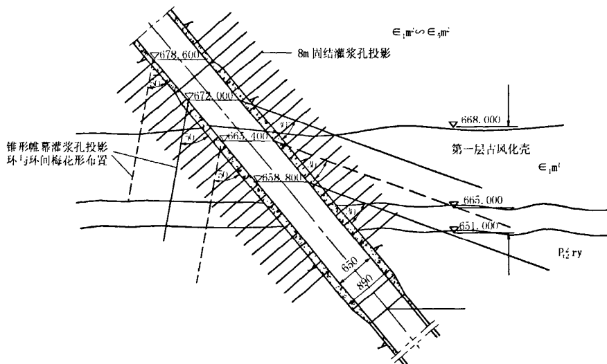
图6 1号引水隧洞上斜井古风化壳部位固结灌浆、锥形帷幕灌浆孔位布置剖面图
