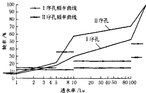
图 2 1 号上斜井帷幕阻水灌浆试验区域 I、II 序孔透水率频率累计曲线图
