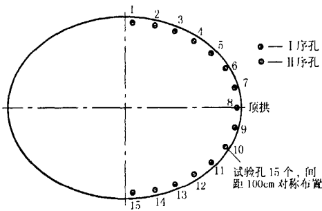
图 1 1 号上斜井帷幕阻水灌浆试验孔位布置图
