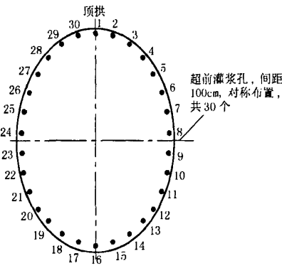
图 4 帷幕阻水灌浆工程第一单元灌浆孔布置图
