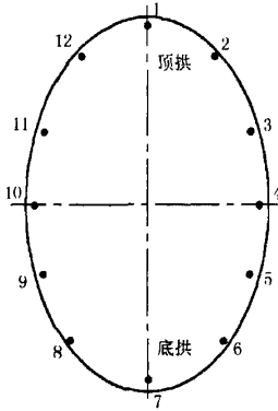
图 5 帷幕阻水灌浆工程第三单元灌浆孔布置图
