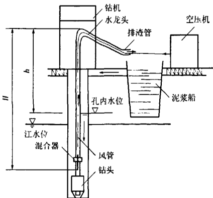
图1 气举反循环示意图
