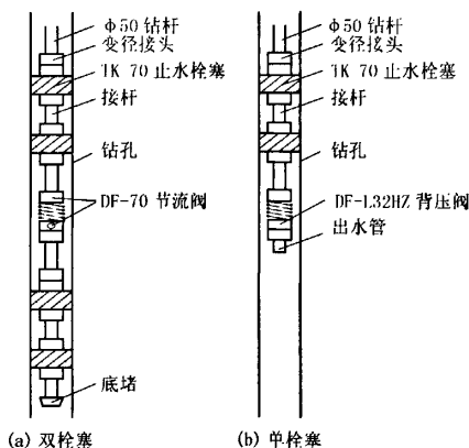
图1 压水器组合示意图
