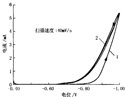
图5 不加氯化铵的镍沉积的循环伏安曲线
