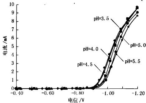
图3 不同 pH 值下的阴极极化曲线
