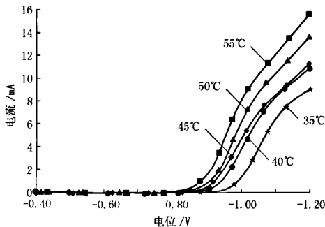
图4 不同温度下的阴极极化曲线
