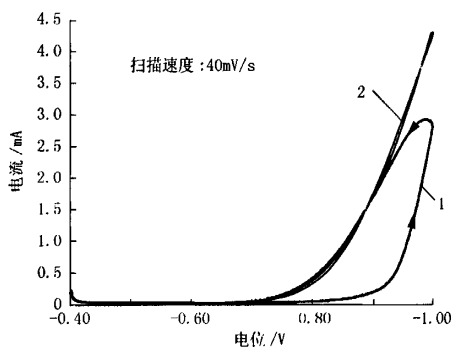
图6 含氯化铵的镍沉积的循环伏安曲线
