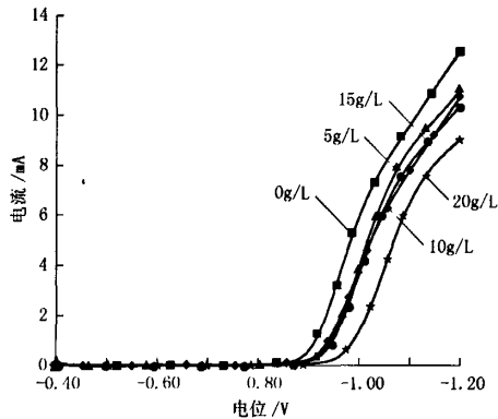
图2 不同 \text{NH}_4\text{Cl} 浓度下的阴极极化曲线
