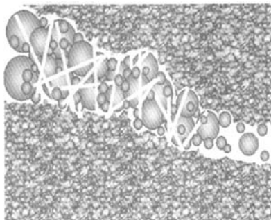
图3 纤维水泥浆堵漏作用原理图
