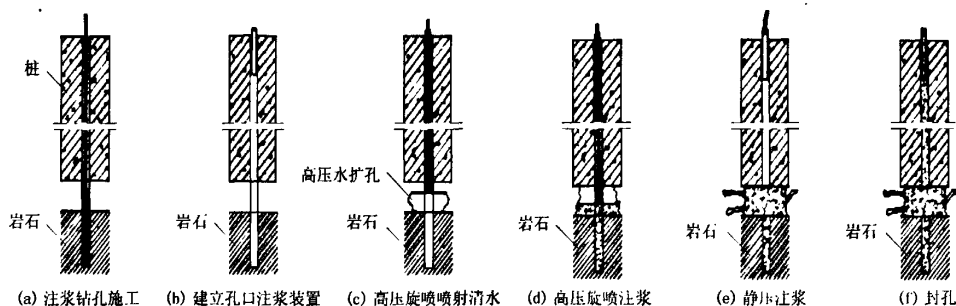
图1 复合注浆加固处理缺陷桩基施工工艺流程
