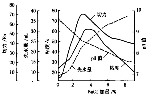
图1 淡水泥浆加 NaCl 后的性能变化
