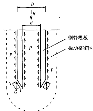
图 1 振动锤配合旋挖钻机施工机理图
