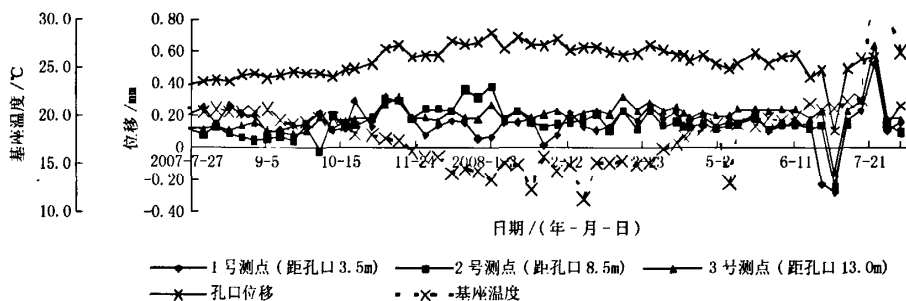
图2 1670 m施工次通道下游边墙K0+160布置的M 4 1多点位移计位移过程曲线
