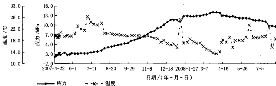
图3 1670 m施工次通道下游边墙K0+160布置的R 1 1锚杆应力计应力变化过程曲线
