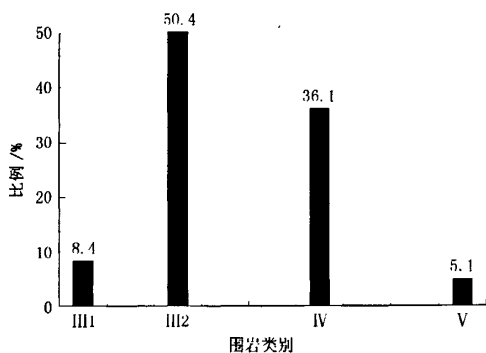
图1 抗力体五层洞室围岩分布统计
